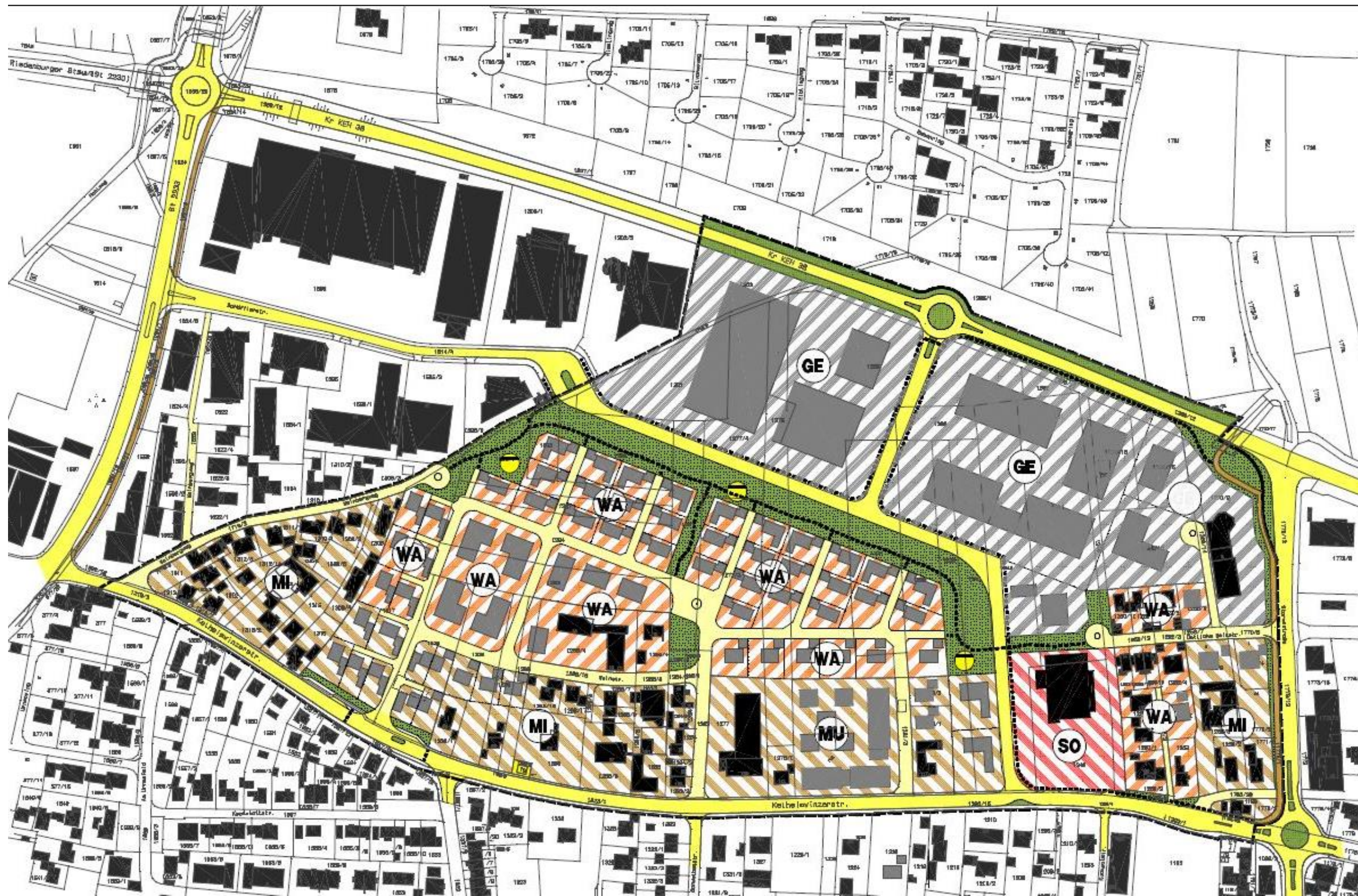
ENTWICKLUNGSKONZEPT (Darstellung unmaßstäblich)
